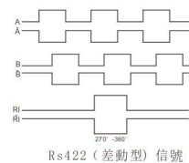
Rs422 (差動型) 信號
