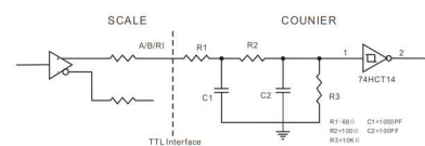
TTL Interface
