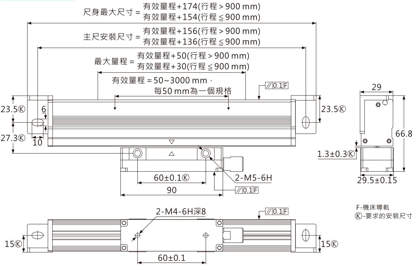
LE安裝尺寸圖
