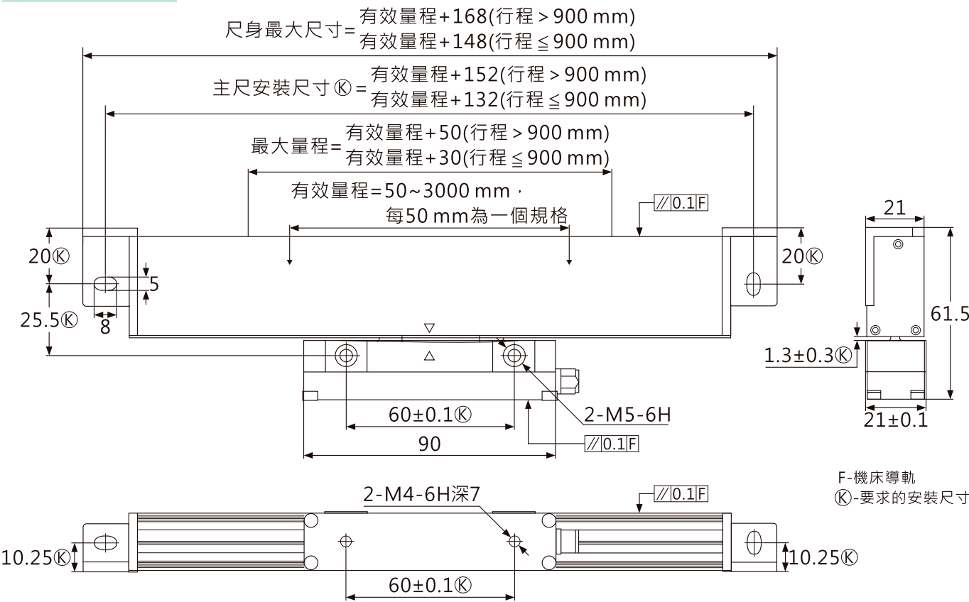
LS安裝尺寸圖
